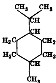
Menthane.
